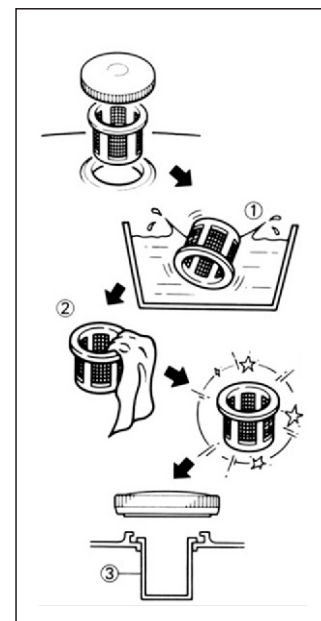
Рисунок 8 – Очистка фильтра топливного бака
